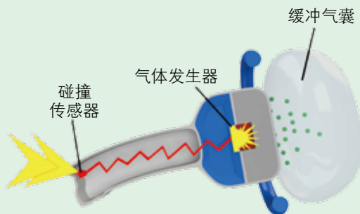
图2-4-5 安全气囊系统示意图
