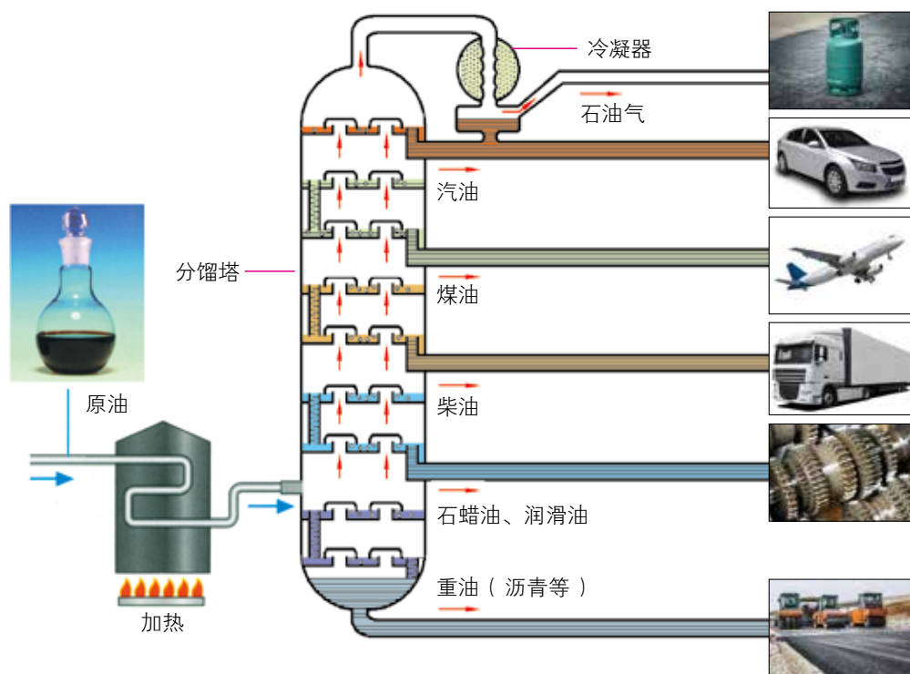
图3-2-6 石油分馏产物及其主要用途
