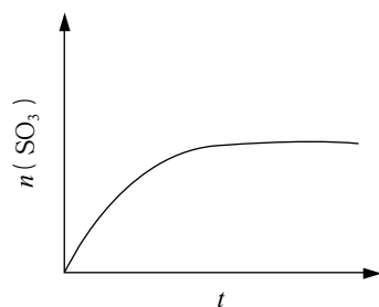
图2-3-6 反应过程中 \text{SO}_3 的物质的量的变化趋势示意图
