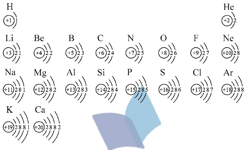
图1-1-5 核电荷数为1~20的元素的原子结构示意图
