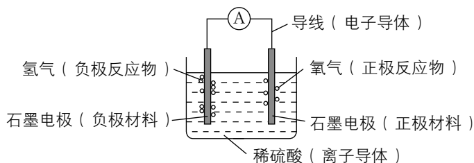
图2-2-10 氢氧燃料电池的构成要素图
