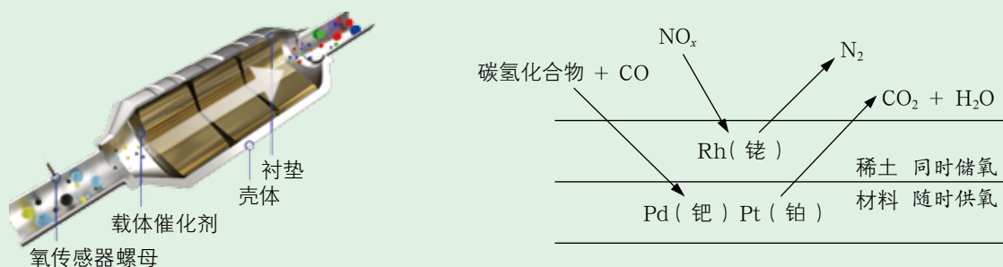
图2-4-4 三元催化器及其工作原理示意图
