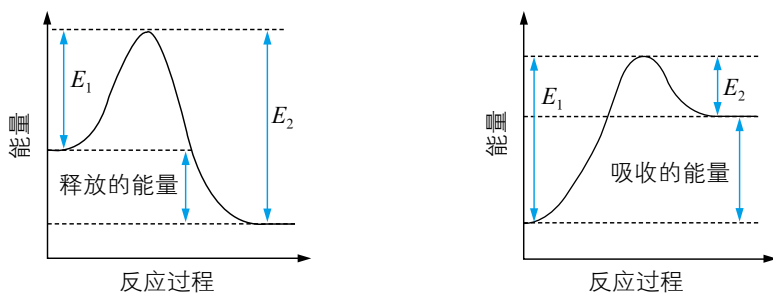
图2-2-5 化学键与化学反应过程中的能量变化
