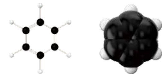
图3-2-10 苯分子的球棍模型和空间填充模型
