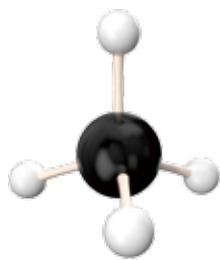
图3-1-3 甲烷分子的球棍模型
