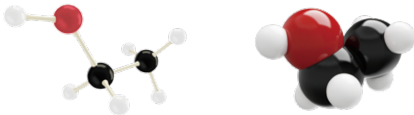
图3-3-2 乙醇分子的球棍模型和空间填充模型
